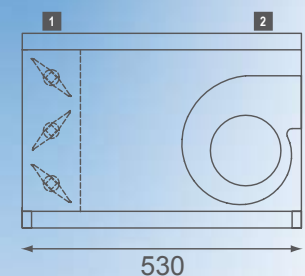
1. Spjæld 2. Ventilator
