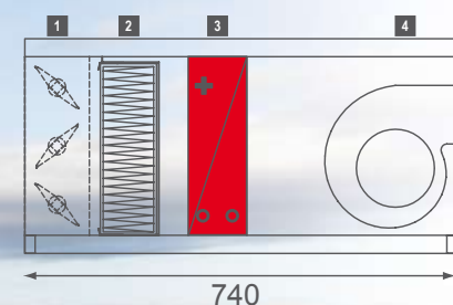
1. Spjæld 2. Filter 3. Varmeflade 4. Ventilator
