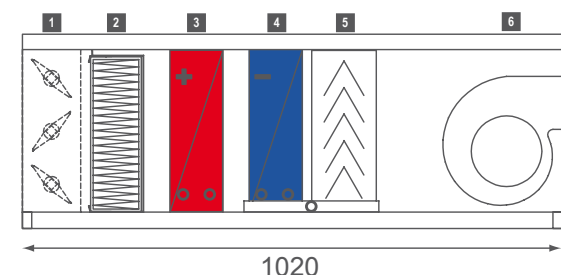
1. Spjæld 2. Filter 3. Varmeflade 4. Køleflade 5. Dråbeudskiller 6. Ventilator
