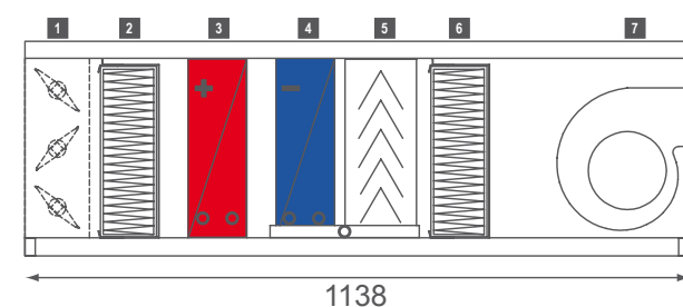
1. Spjæld 2. Filter F5 3. Varmeflade 4. Køleflade 5. Dråbeudskiller 6. Filter F7 7. Ventilator
